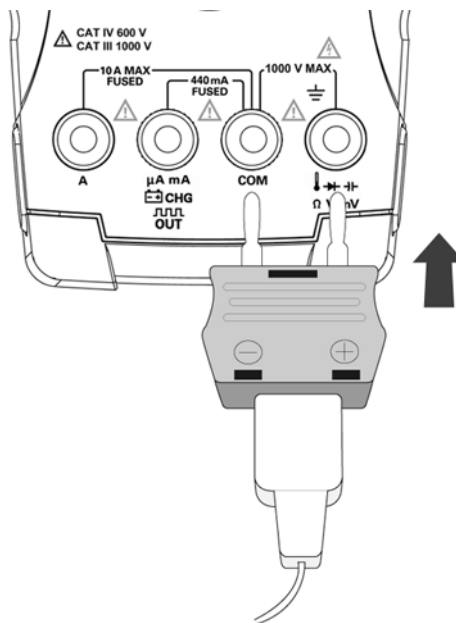
圖 2-16 將連接了配接器的探頭連接到萬用電表
