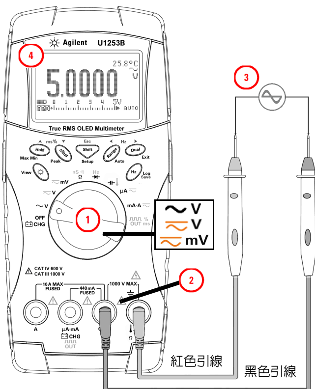
圖 2-1 量測 AC 電壓
