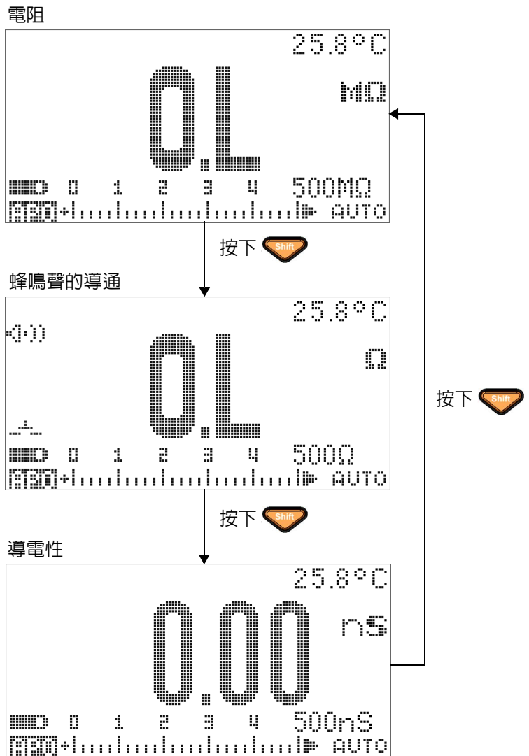
圖 2-9 電阻、蜂鳴聲的導通和導電性測試
