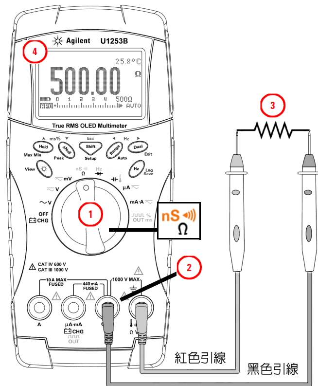
圖 2-8 量測電阻
