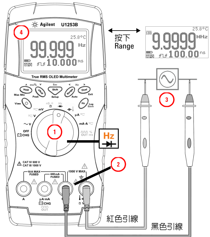
圖 2-6 量測頻率
