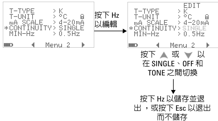
圖 4-10 選擇用於導通測試的聲音
