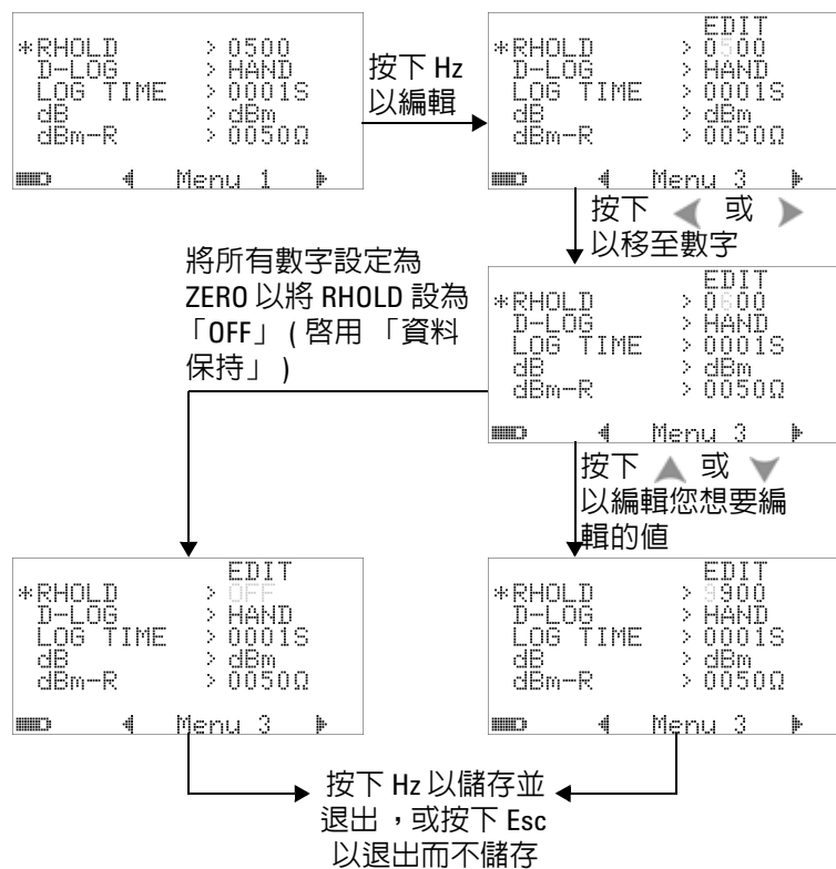
圖 4-2 資料保持 / 重新整理保持設定
