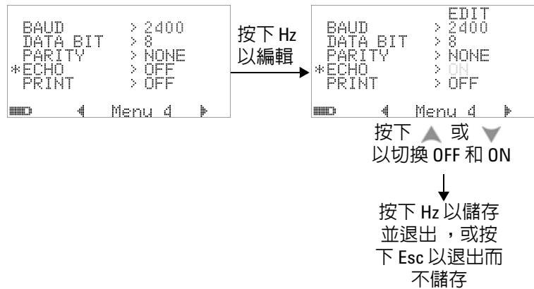
圖 4-20 為遠端控制設定回應模式
