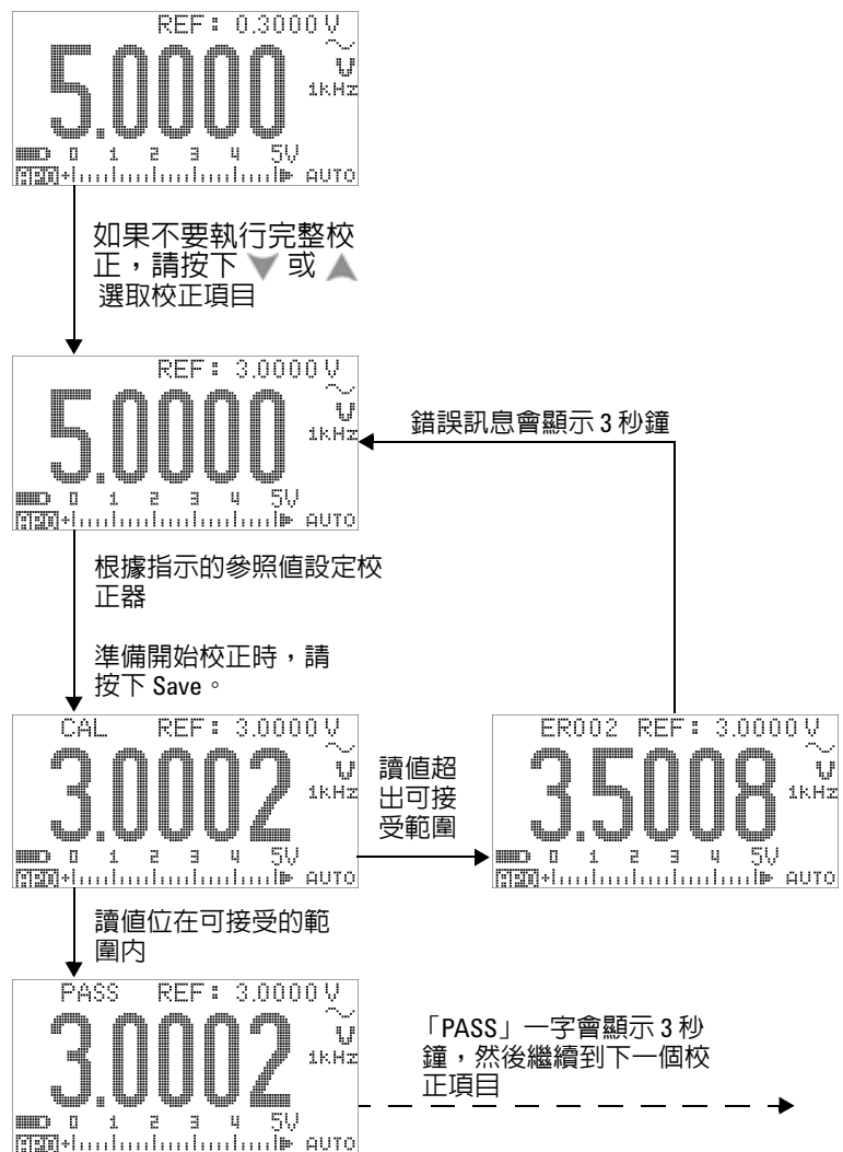
圖 6-7 一般校正程序流程
