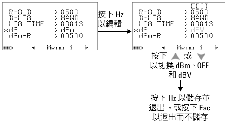
圖 4-5 分貝量測設定
