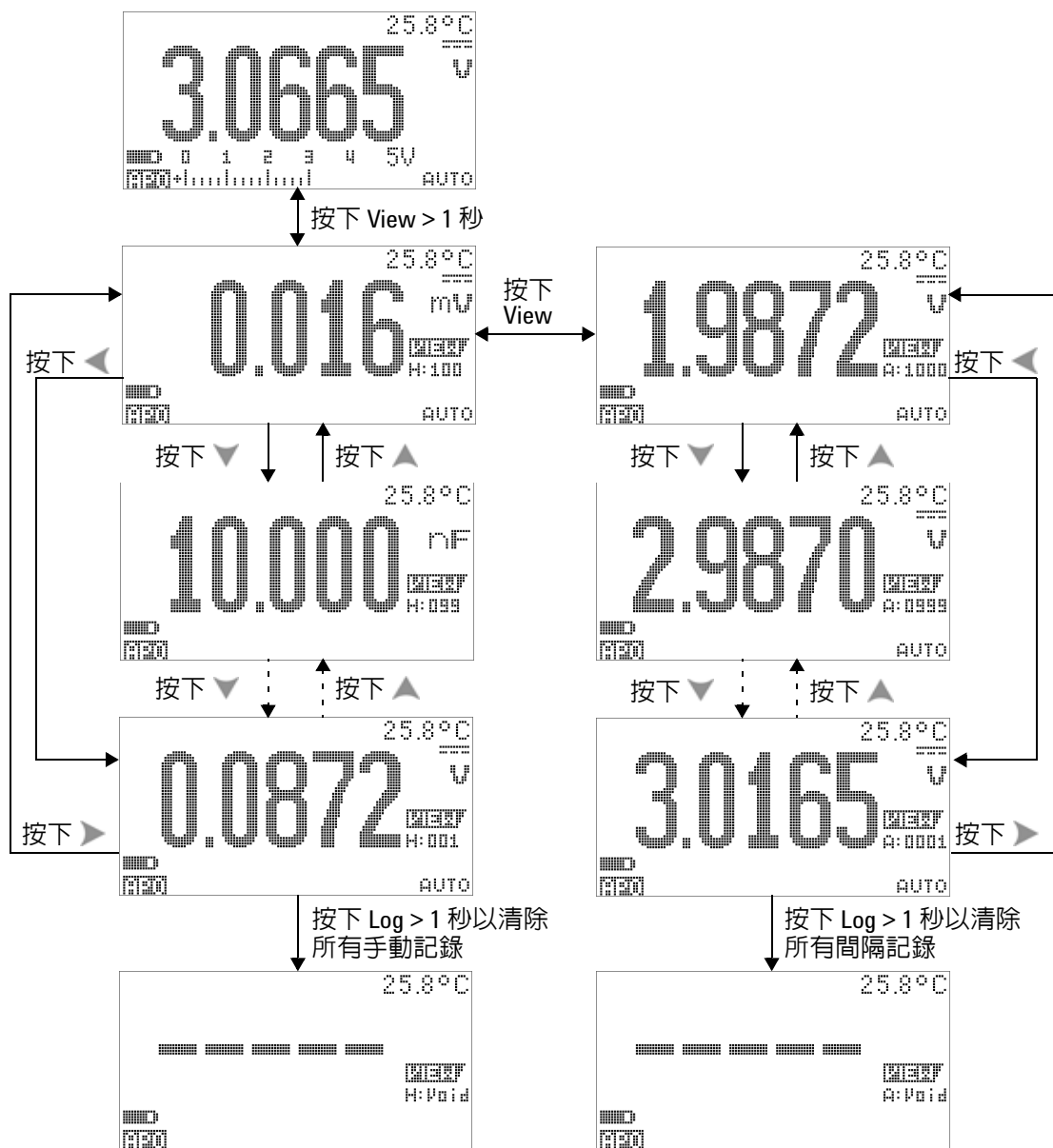
圖 3-11 記錄檢閱模式操作
