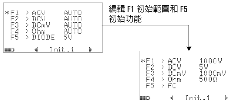
圖 4-27 編輯初始量測功能 / 範圍
