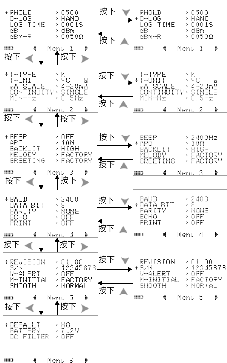
圖 4-1 設定功能表畫面
