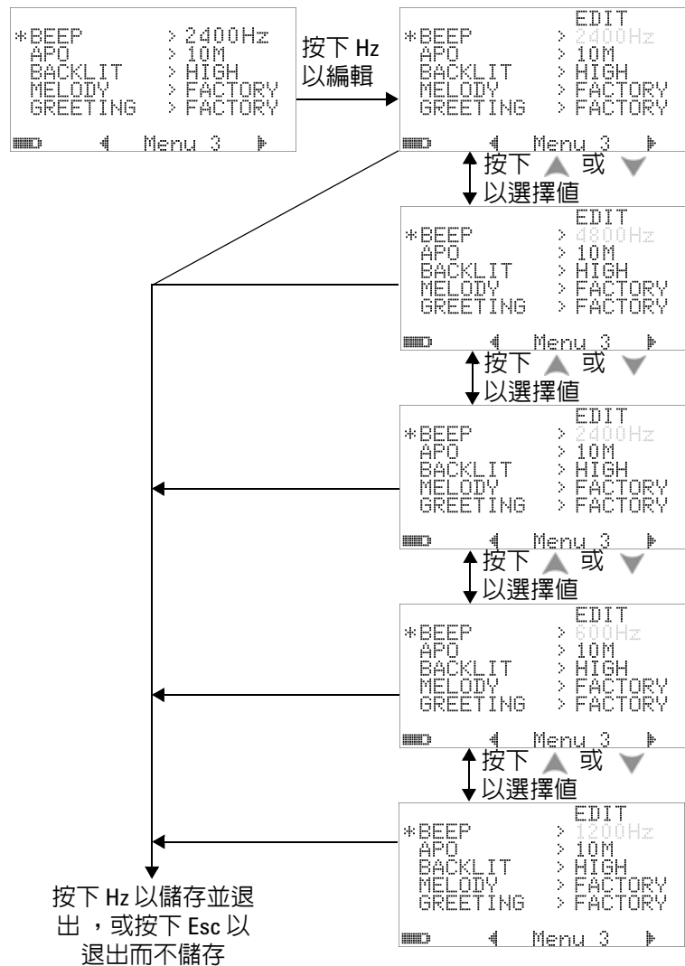
圖 4-12 嗶聲頻率設定
