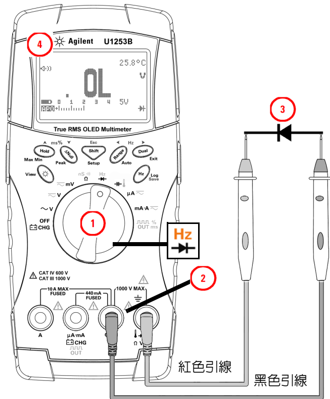
圖 2-13 量測二極體的逆向偏壓
