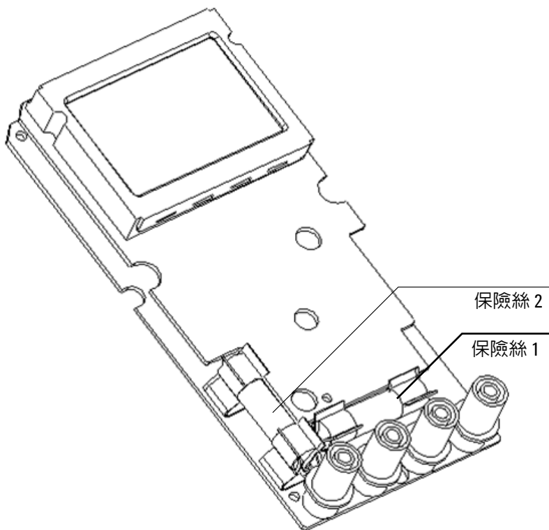
圖 5-9 更換保險絲
