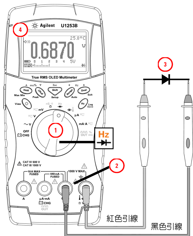
圖 2-12 量測二極體的順向偏壓
