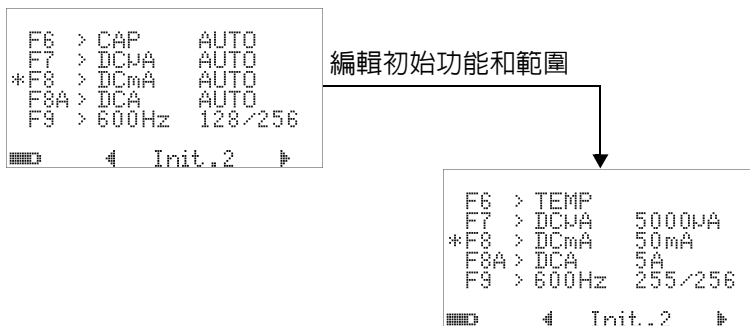
圖 4-28 編輯初始量測功能 / 範圍和初始輸出值
