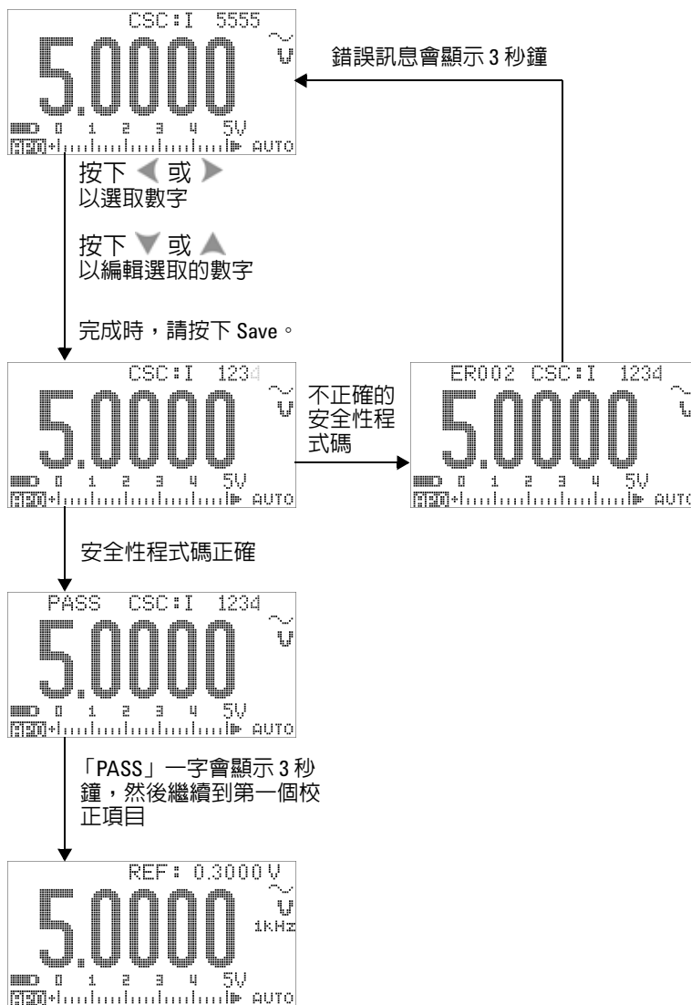
圖 6-4 解除保護儀器以進行校正
