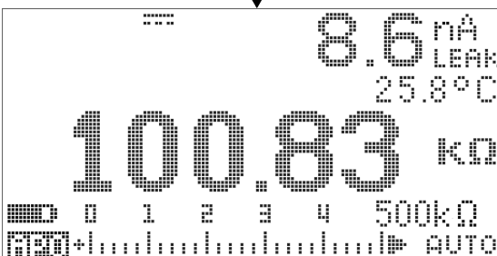
圖 2-7 啓用 Smart \Omega 時的顯示類型
