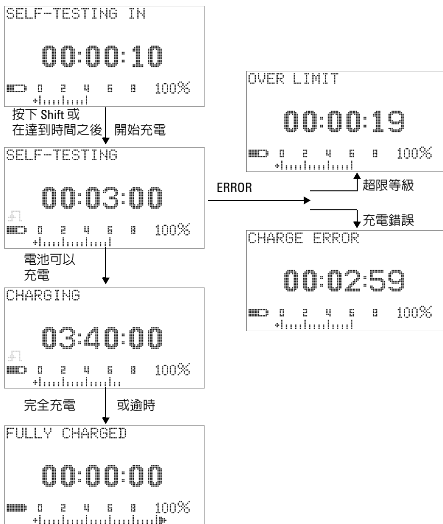
圖 5-7 電池充電程序
