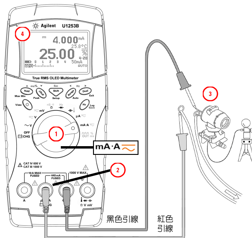
圖 2-4 4 mA 到 20 mA 的量測標度
