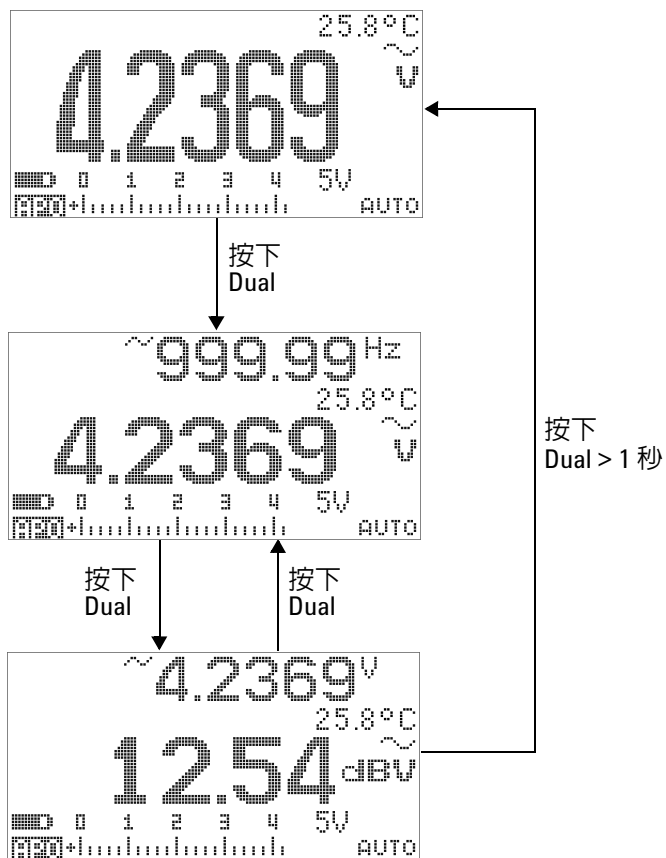
圖 3-6 dBV 顯示器模式操作
