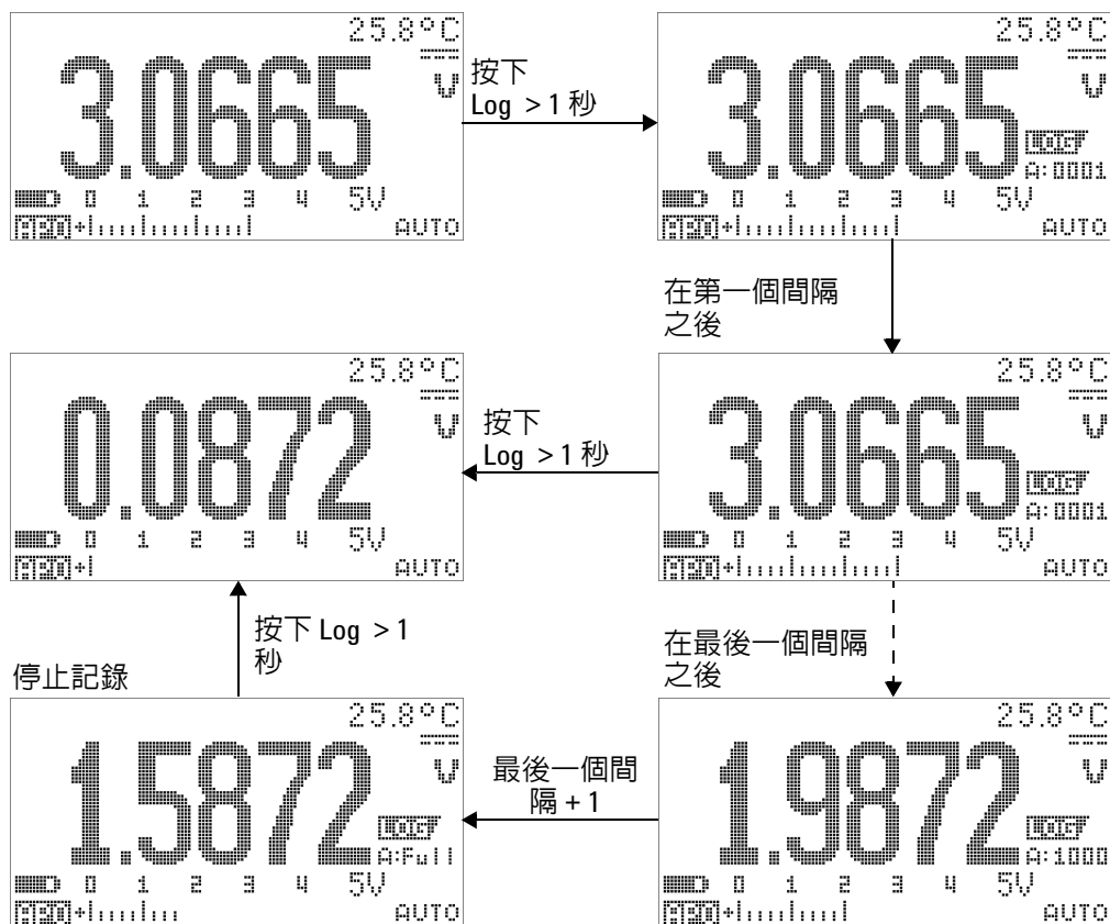
圖 3-10 間隔 (時間) 記錄模式操作
