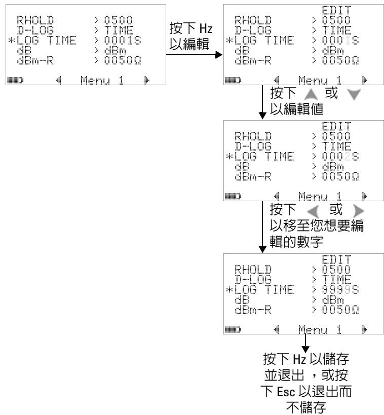
圖 4-4 間隔 (時間) 記錄的記錄時間設定
