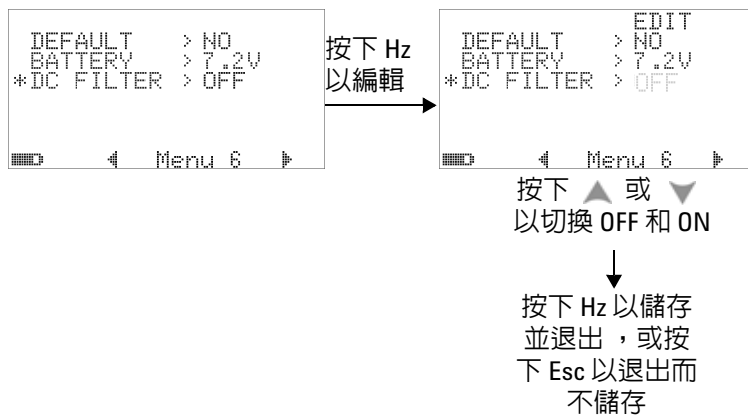
圖 4-32 DC 濾波器
