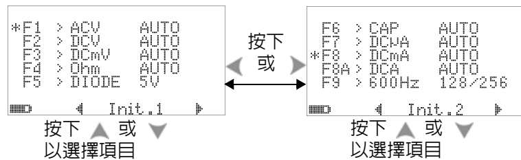
圖 4-26 瀏覽初始功能頁面
