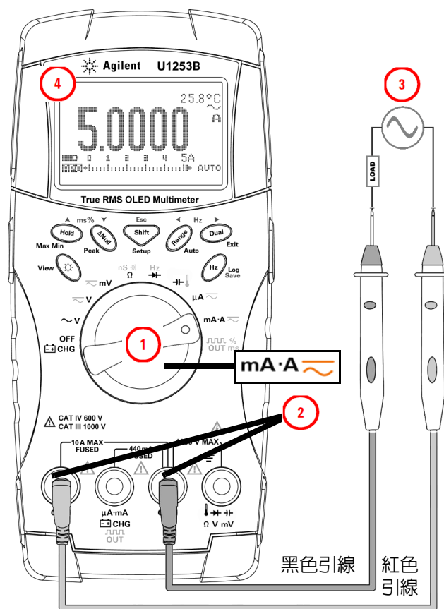
圖 2-5 A (安培) 電流量測
