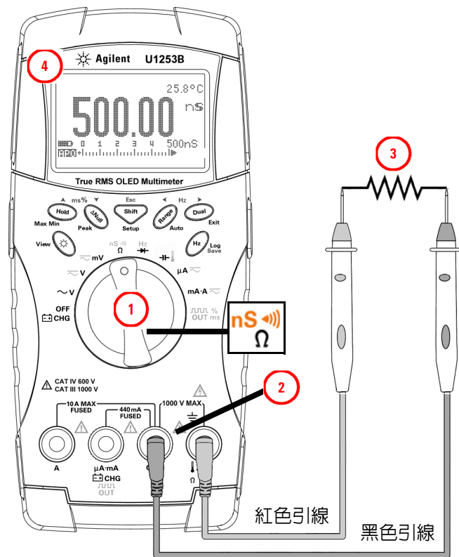
圖 2-11 導電性量測
