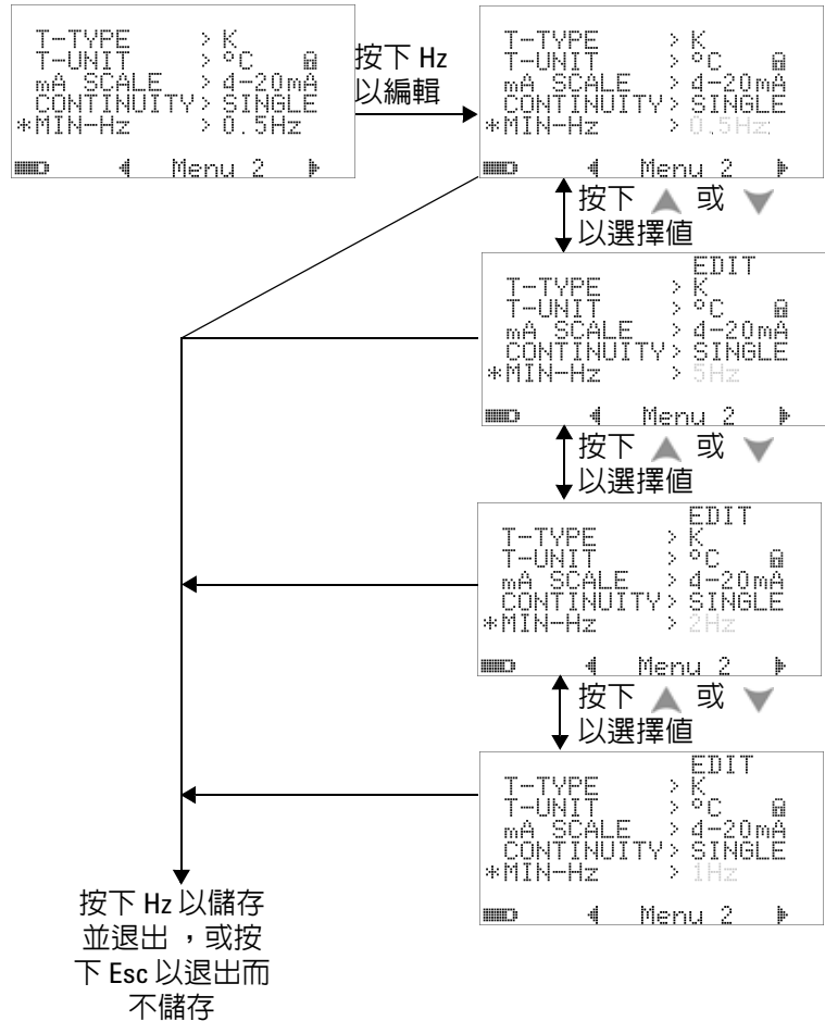
圖 4-11 最小頻率設定
