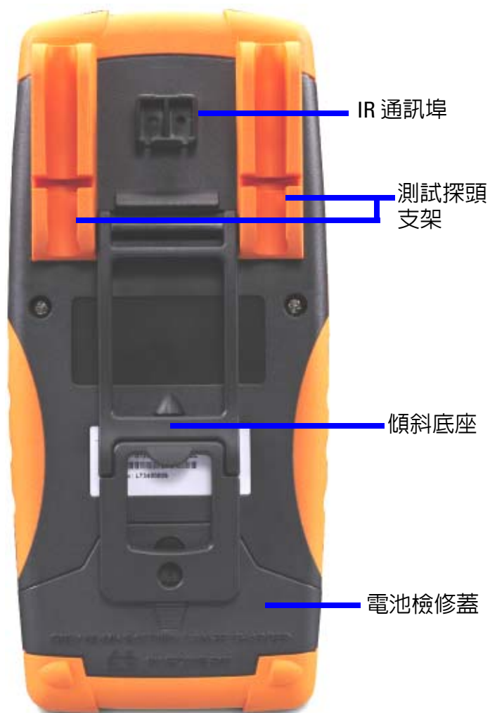
圖 1-5 U1253B 的後端面板
