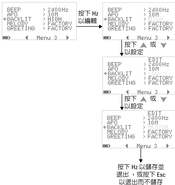
圖 4-14 開機背光設定
