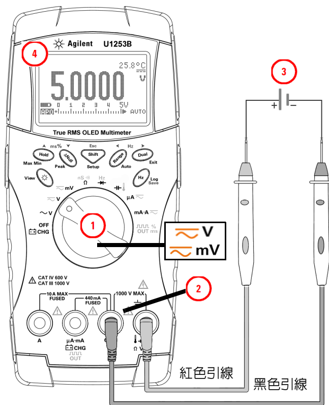
圖 2-2 量測 DC 電壓
