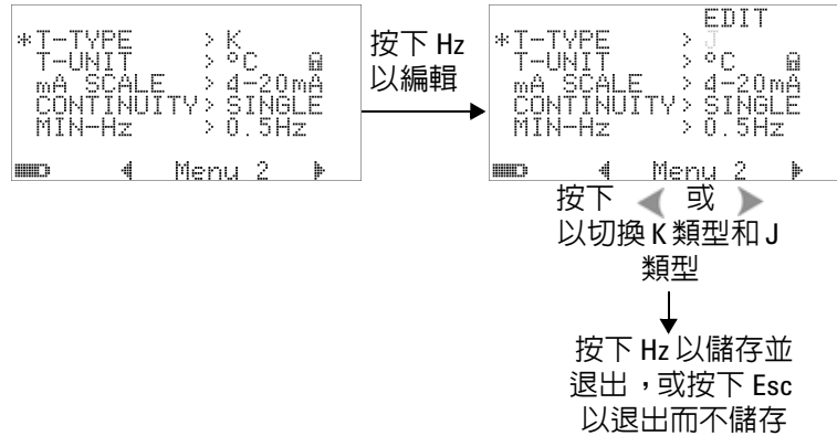
圖 4-7 熱耦合類型設定
