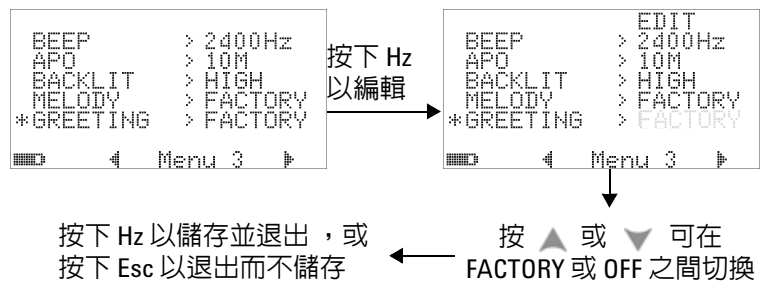
圖 4-16 開機問候設定
