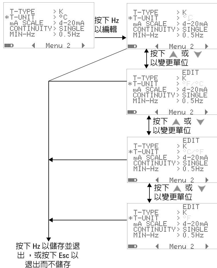
圖 4-8 溫度單位設定
