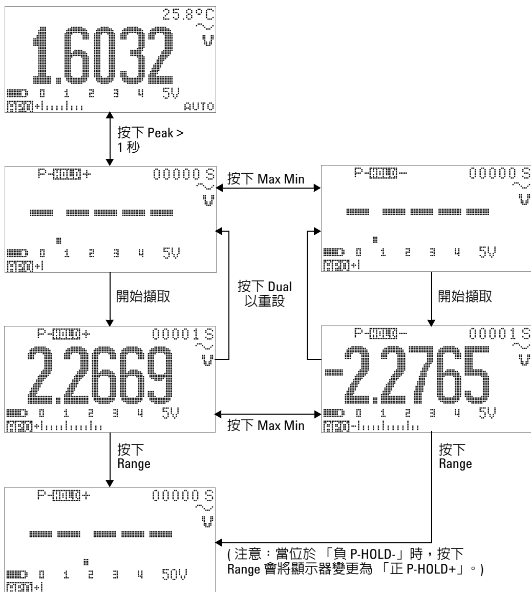
圖 3-7 1 ms 峰值保持模式操作
