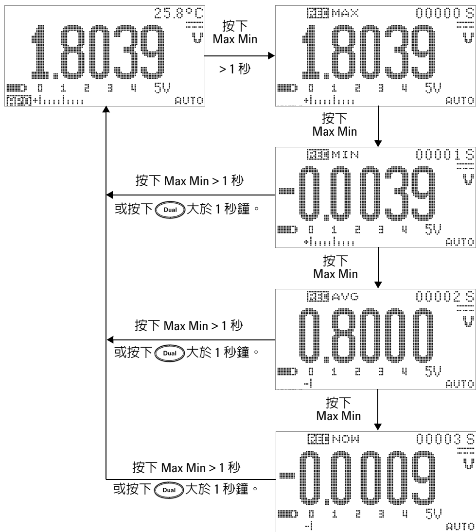
圖 3-1 動態記錄模式操作
