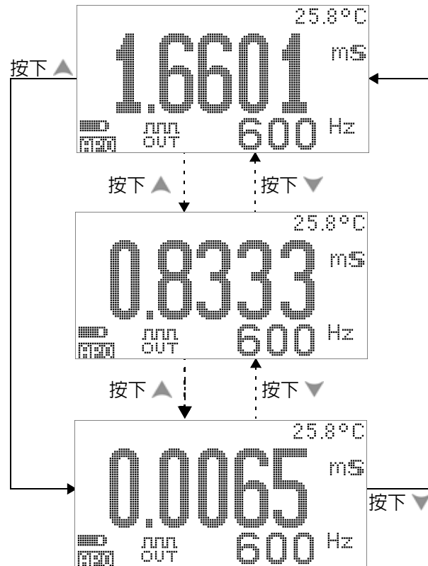
圖 3-14 方波輸出的脈衝寬調整
