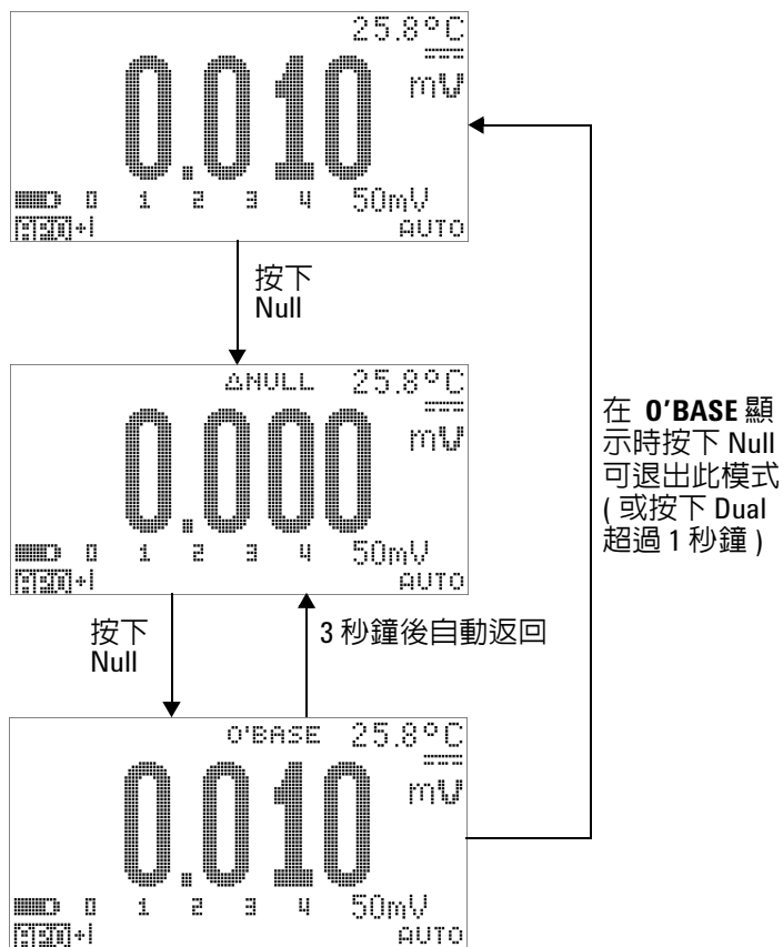
圖 3-4 Null (相對) 模式操作
