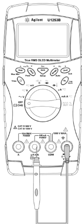
圖 5-8 保險絲檢查過程
