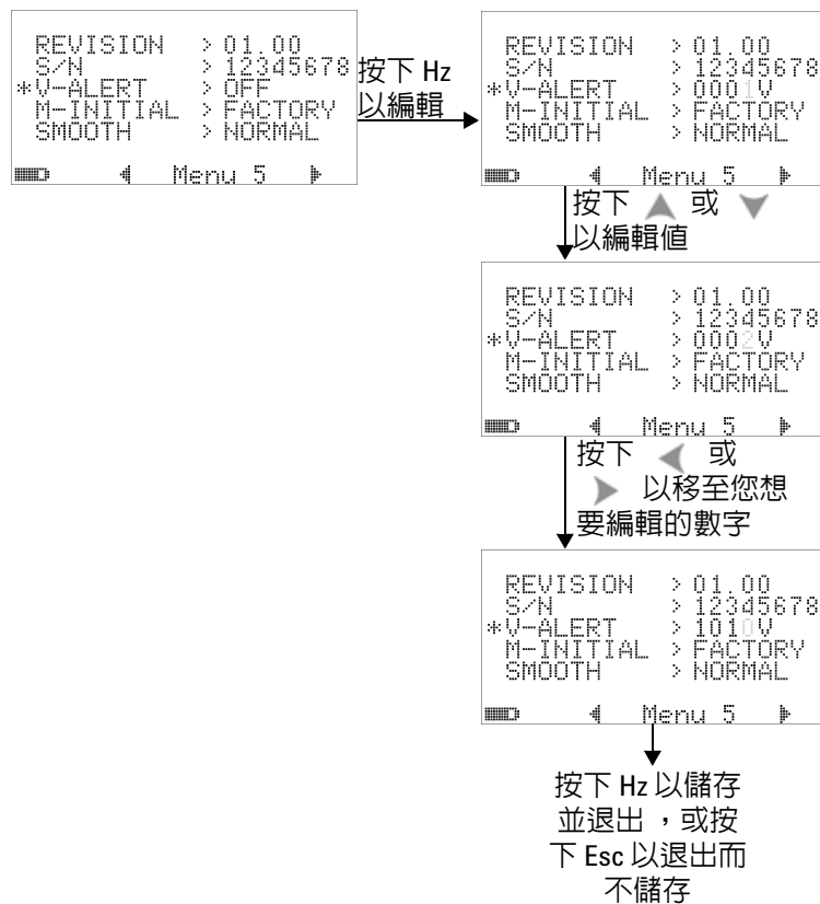
圖 4-24 電壓警示設定
