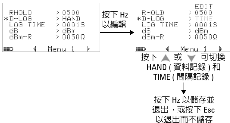
圖 4-3 資料記錄設定
