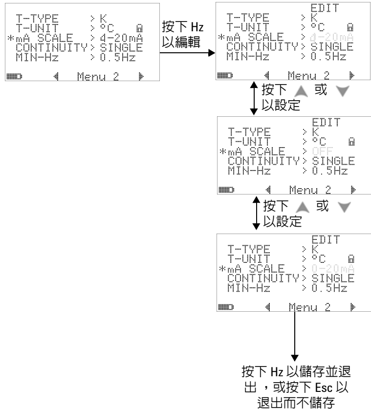
圖 4-9 設定百分比標度讀數
