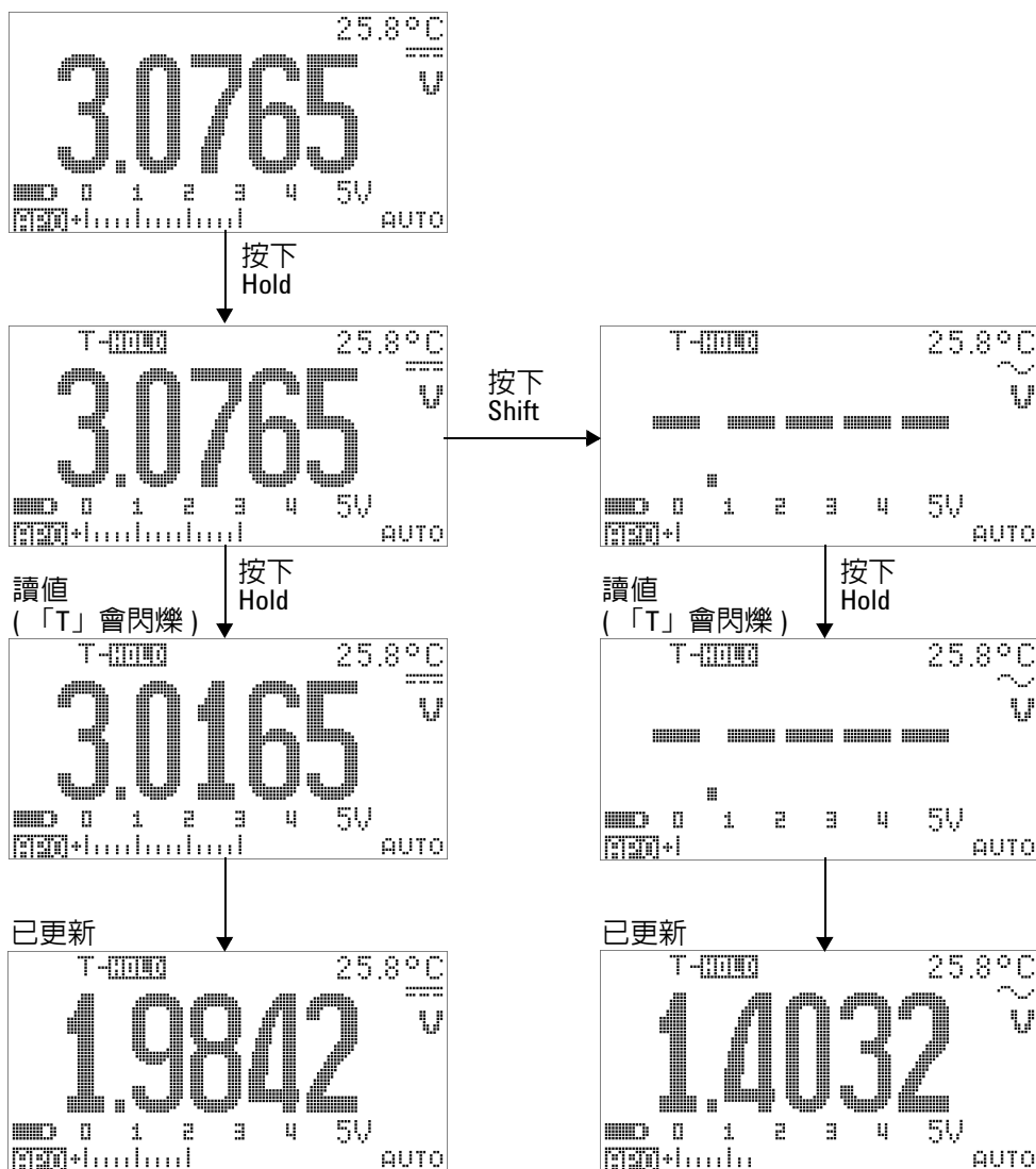
圖 3-2 資料保持模式操作
