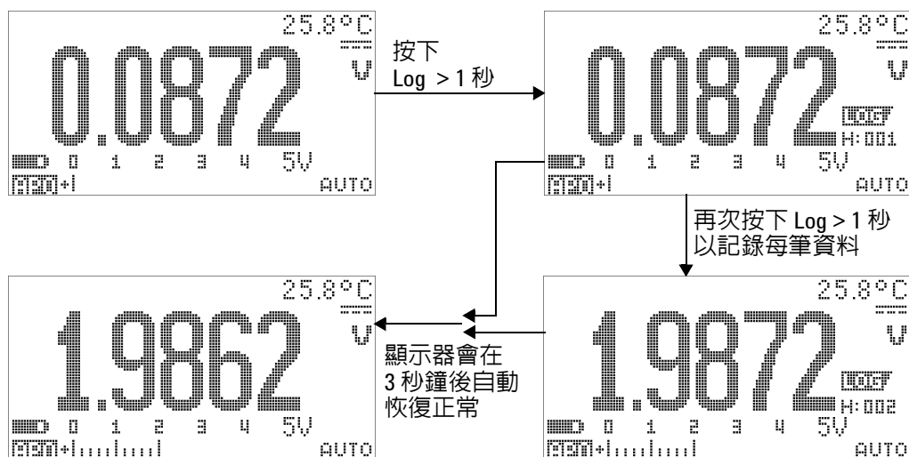
圖 3-8 手動（手）記錄模式操作
