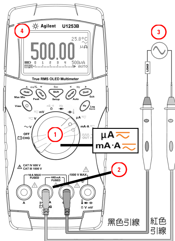
圖 2-3 量測 \mu\text{A} 和 mA 電流
