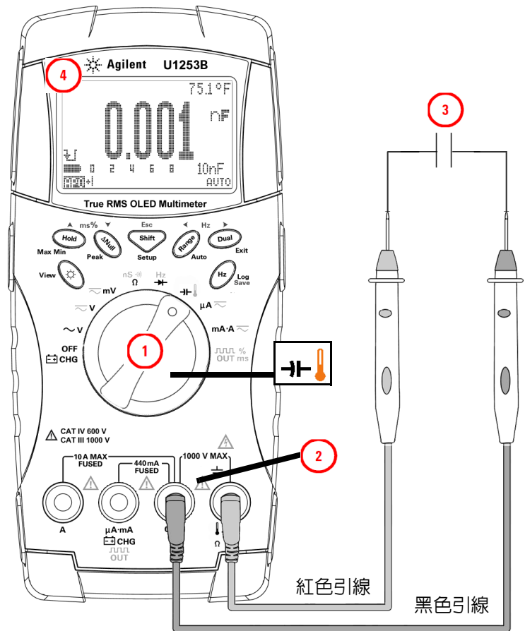
圖 2-14 電容量測
