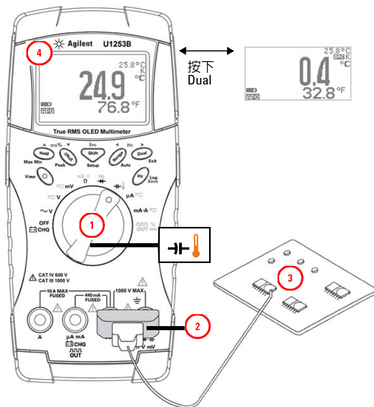
圖 2-17 表面溫度量測
