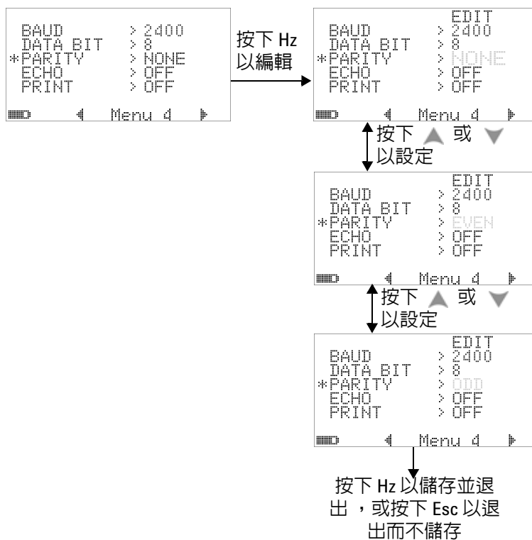
圖 4-19 為遠端控制設定同位檢查
