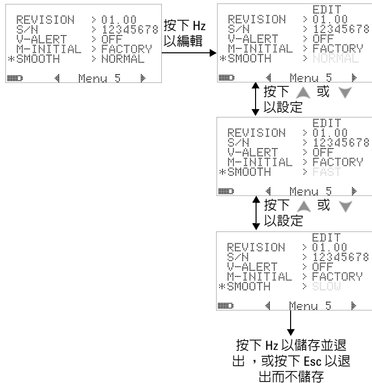
圖 4-29 主要顯示器讀值的重新整理速率
