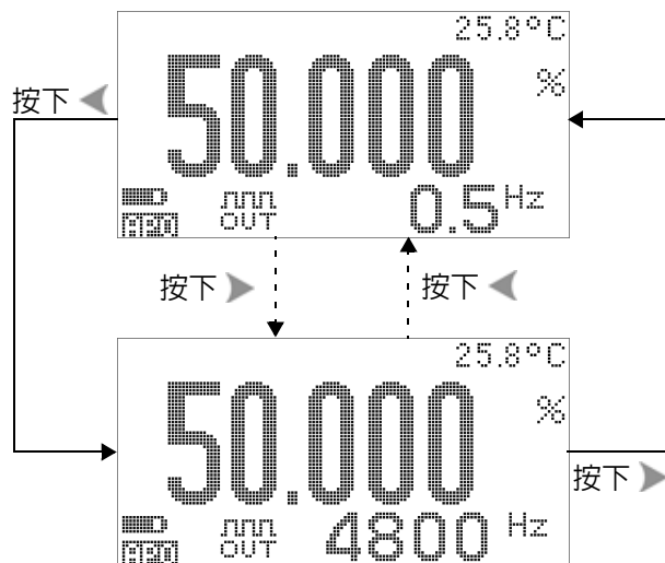
圖 3-12 方波輸出的頻率調整
